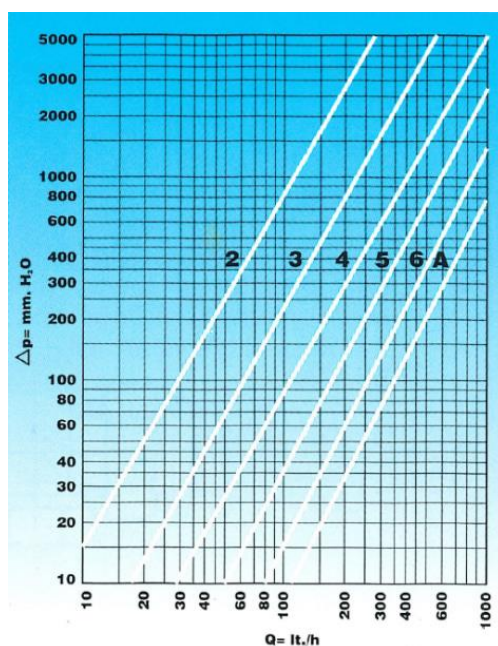
Detentore dritto
